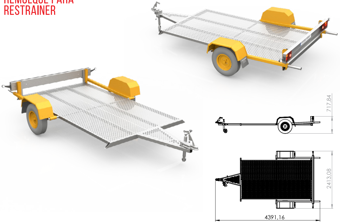
B376 RESTRAINER OVINO CON REMOLQUE
